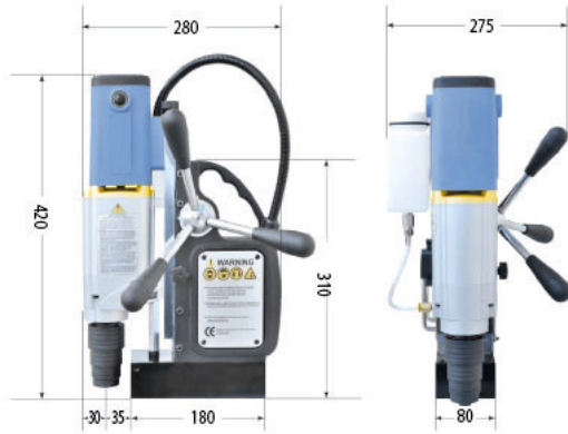
MAGPRO TP 2000
